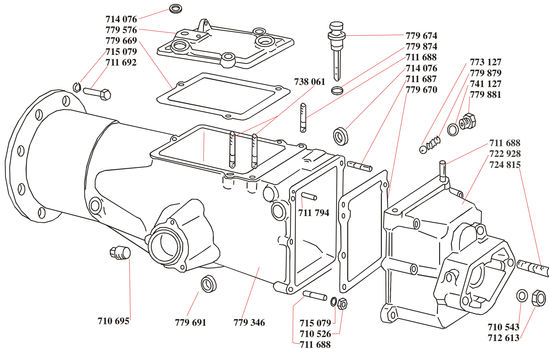
OHIŠJE Z DIFERENCIALOM
